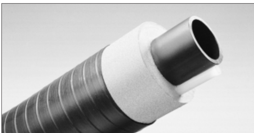
Isovarm 110/200 mm PE 50 PN 10 med tomrör för värmekabel
